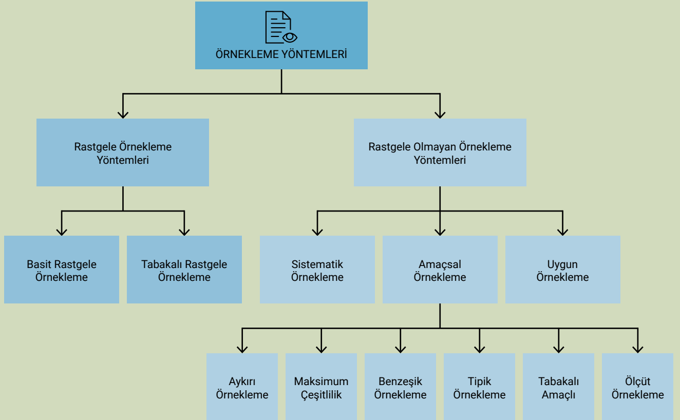
Şekil 27: Örnekleme Yöntemleri
